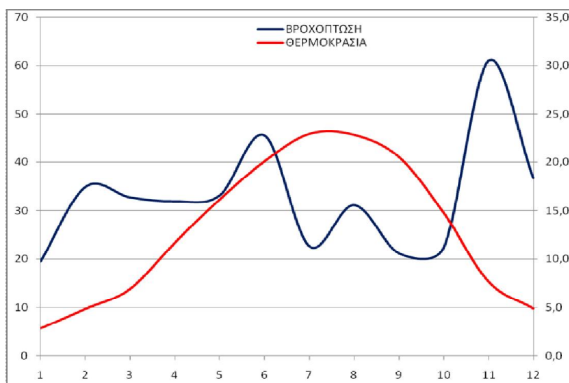
Διάγραμμα 1. Ομβροθερμικό διάγραμμα περιοχής ευθύνης Δασαρχείου Κιλκίς.
